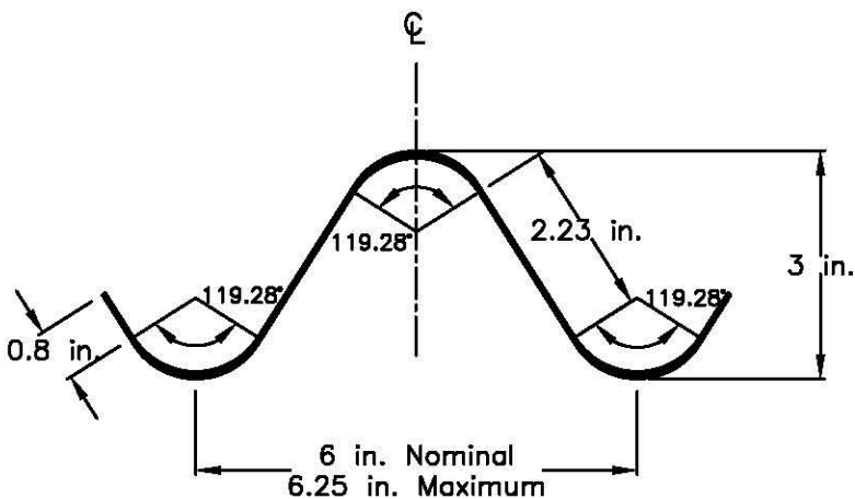
FIG. 1 TYPE 1 RIB STIFFENER
