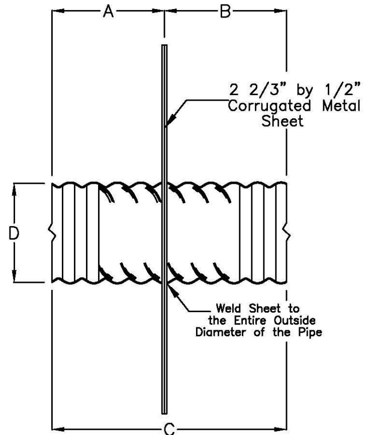
SECTION A-A
